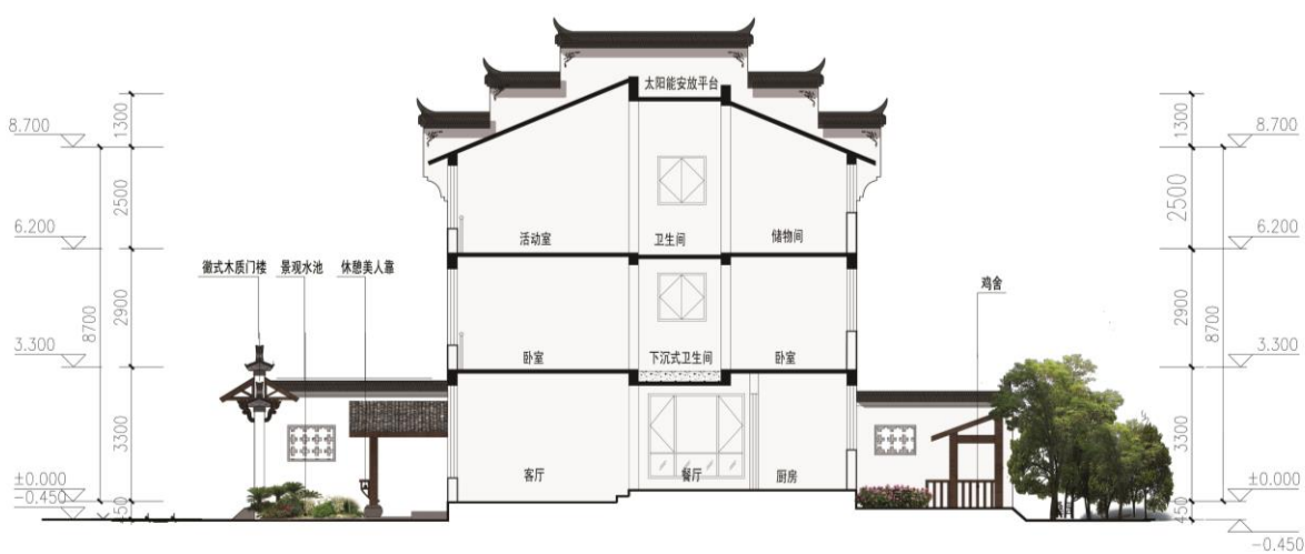
剖面图
